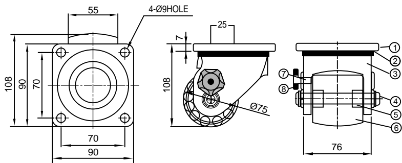
WIM- 800FP(F) TYPE
